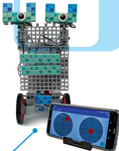
Робот "Наум"
